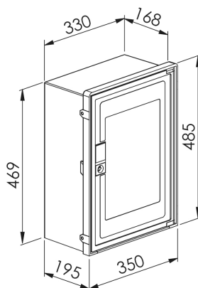
Schéma coffret S20
