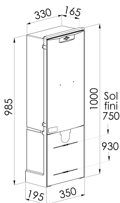
Schéma borne ECP2D
