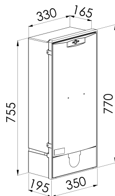
Schéma coffret ECP2D
