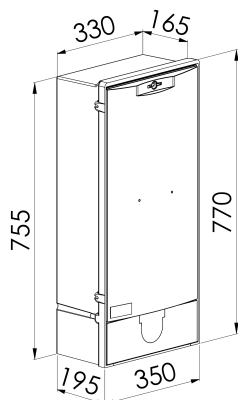
Schéma coffret REMBT 300
