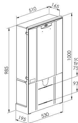
Schéma borne REMBT 450
