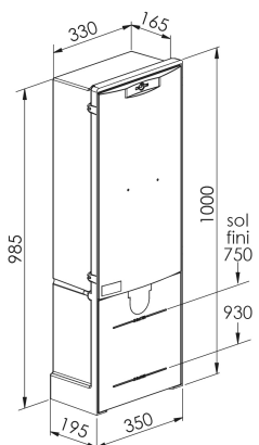
Schéma borne REMBT 300
